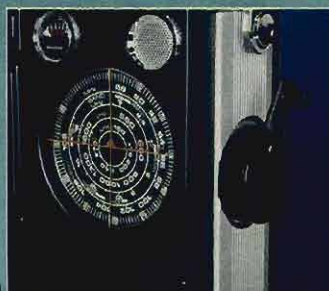
1. Neu: Kombinierte Aufnahme-/VAT-Taste für stufenloses Ein- und Ausblenden bei jeder Aufnahme 2. Bedienungs-Deck mit Bereichs- und Betriebsarten-Schaltern 3. Kurbel des Abstimmknopfes für Quicktuning herausgeklappt 4. Abstimm-Instrument mit Batterie-/Accu-Anzeige kombiniert 5. Gehäuseausführung schwarz Profi-Look
